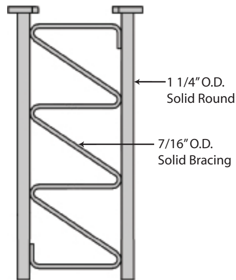
4.3' 45GSR SHORT BASE 45GSRSB
