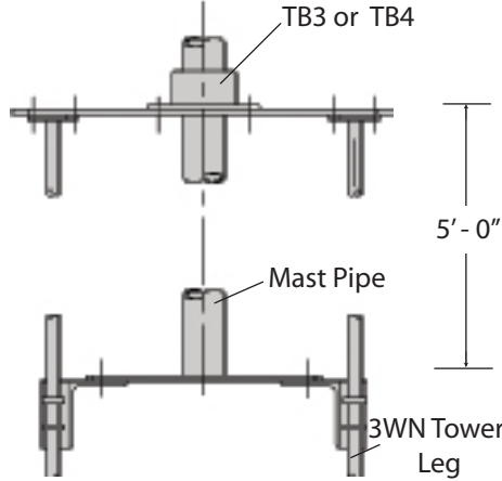
P/N: VU474A
