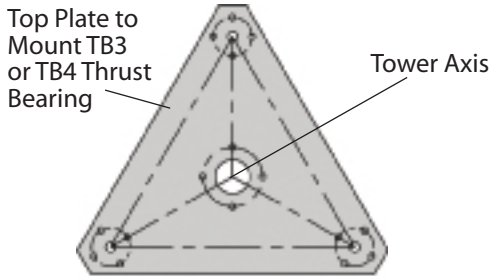
1W / 2W
